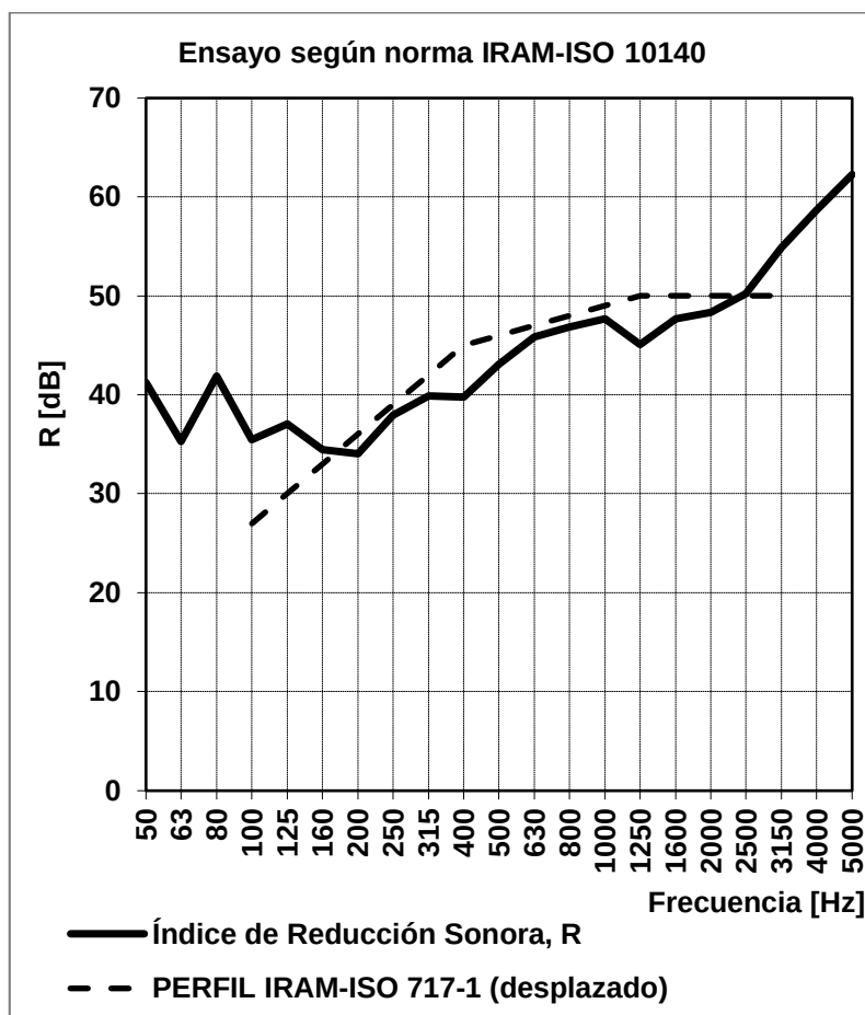
Gráfico 1: Índice de reducción sonora R
