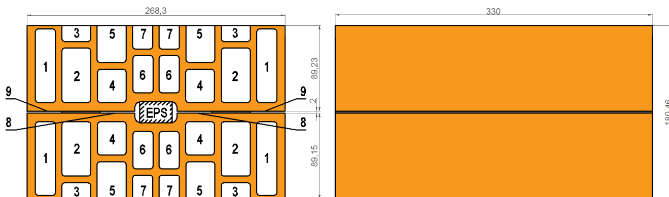
Corte transversal
